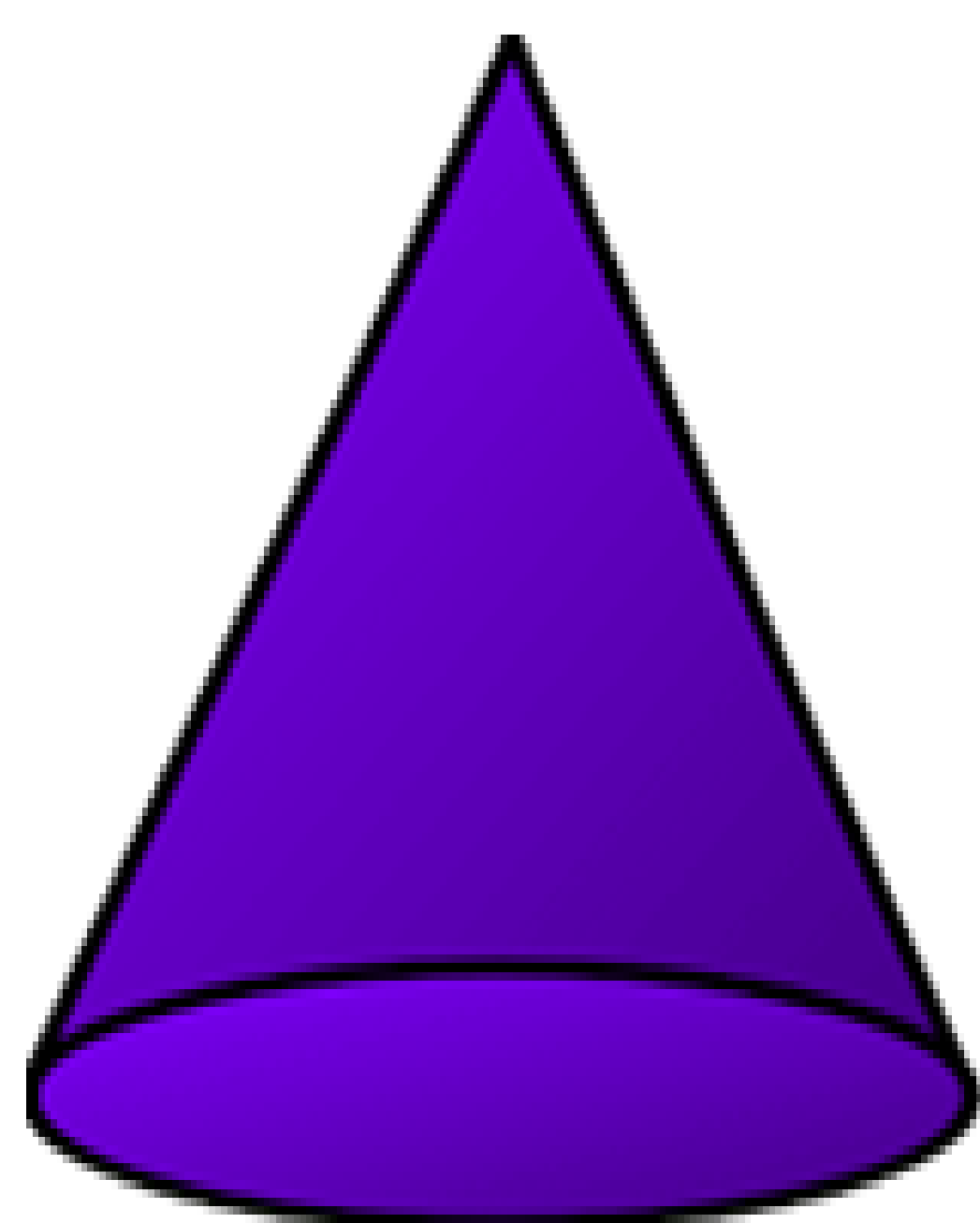
Cone
